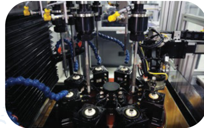
Máy mài lỗ Bore - Honing
